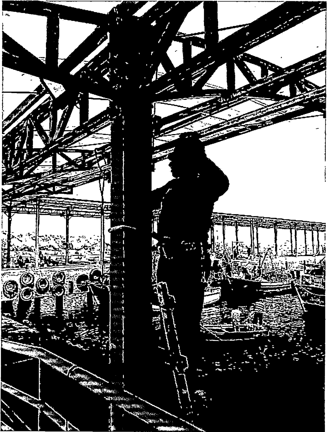
Fotografía N°07: Vista de instalación de tuberías Conduit en muelle 1.
