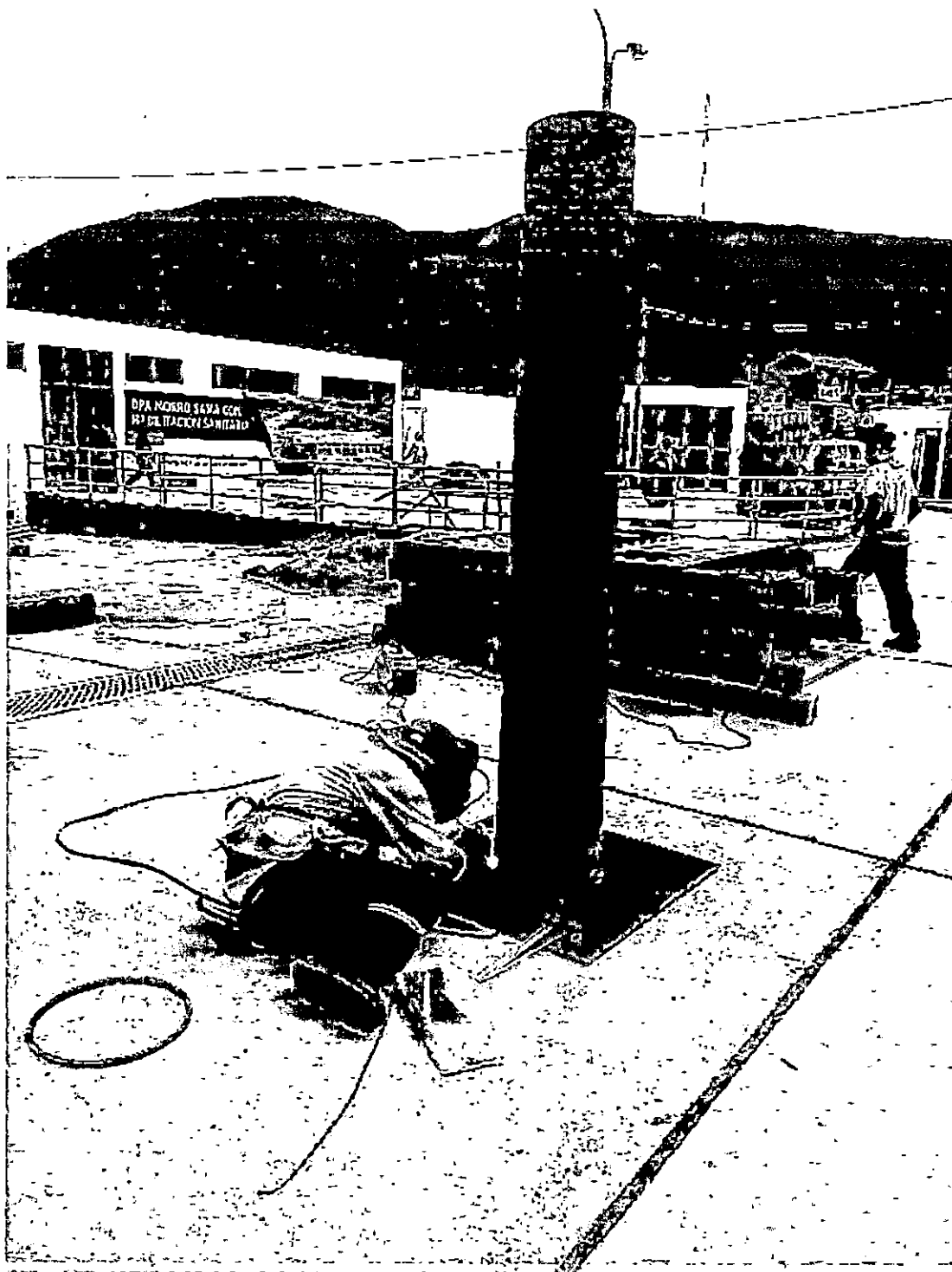
Fotografía N°12: Vista de base metálica para poste de fibra de vidrio.
